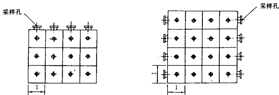
图 6 长方形断面的测定点
