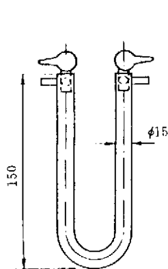
图 12 重量法测定排气水分含量装置
