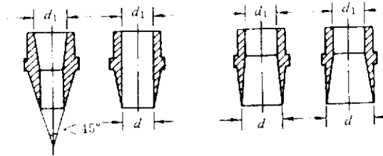
图 22 采样嘴
