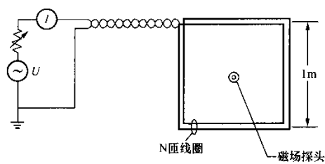
图 B.5 磁场仪校准布置图
