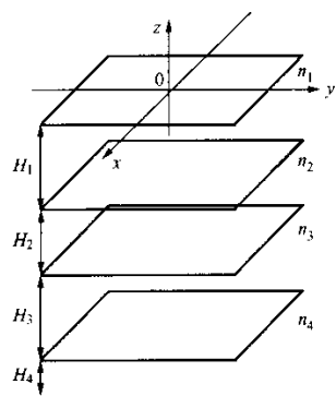
图 B.2 线圈排列举例
