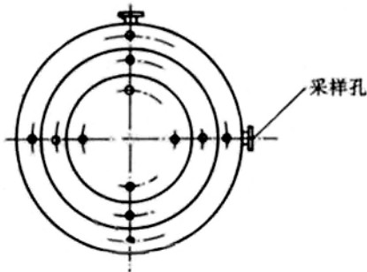
图 3 圆形断面的测定点
