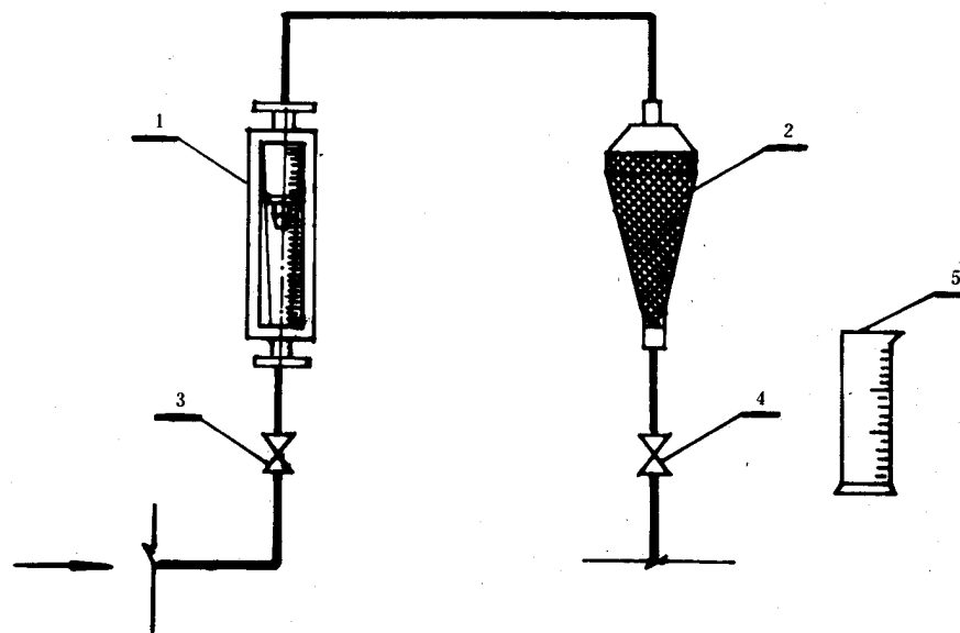
1—转子流量计;2—浮游生物网;3—J11X-10 截止阀; 4—X43W-10 旋塞阀;5—量筒
