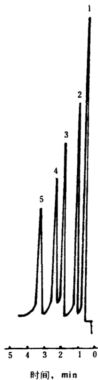
图 B1 用热解吸法色谱图 1 苯；2 甲苯；3 对、间二甲苯； 4 邻二甲苯；5 苯乙烯
