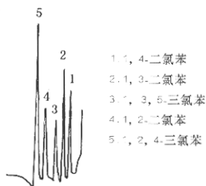
图 1 氯苯类化合物的气相色谱图
