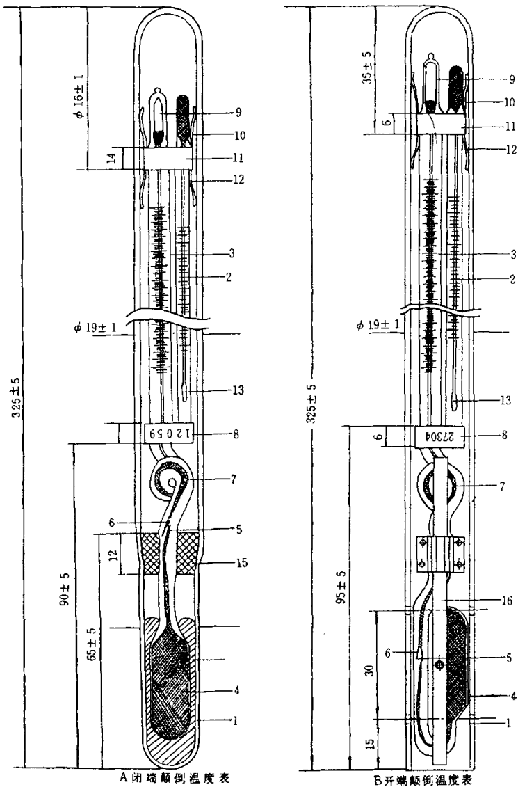
1—外套管；2—副温度表；3—主温度表；4—主温度表贮蓄泡；5—盲枝；6—断点；7—圆环； 8—出厂编号及卡箍；9—主温度表接收泡；10—副温度表贮蓄泡；11—卡箍；12—弹簧片； 13—付温度表安全泡；14—水银槽；15—软木塞；16—开端颠倒温度表椭圆弹簧键
