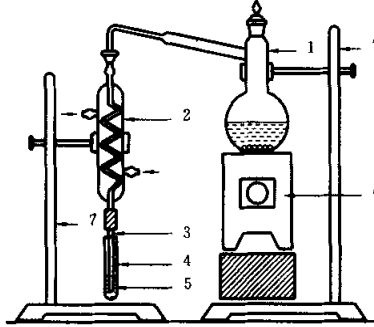
1—1 升全玻璃磨口蒸馏瓶; 2—蛇形冷凝管; 3—玻璃管; 4—50 mL 具塞比色管; 5—氢氧化钠吸收液; 6—万用电炉; 7—铁架台
