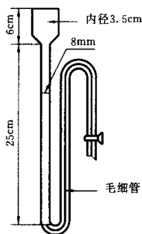
图 21 还原柱
