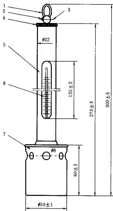
1—提环；2—销钉；3—开口销；4—帽头；5—表管；6—温度表；7—贮水筒
