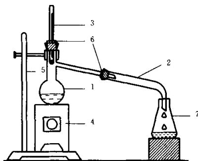
1—10 或 25 mm 微量蒸馏烧瓶;2—空气冷凝管;3—250℃水银温度计;4—电炉; 5—铁架台;6—软木塞;7—三角烧瓶(收集苯酚)
