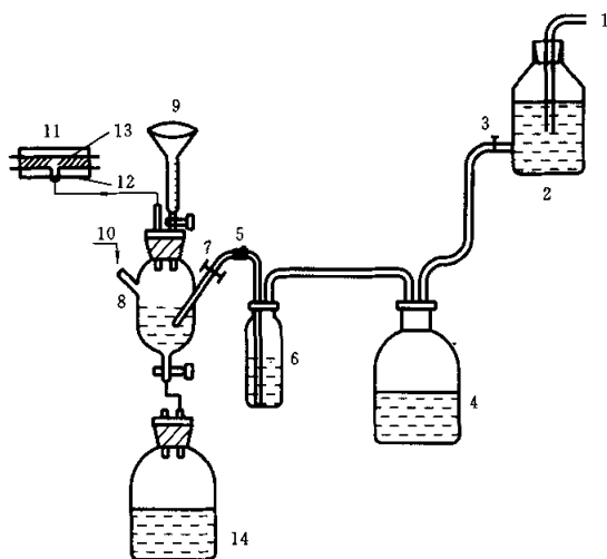
1—马利奥特管；2—水槽；3—阀门；4—接水瓶；5—流速控制管；6—KBH 4 瓶；7—弹簧夹；8—反应瓶；9—进液漏斗； 10—N 2 或Ar进口；11—吸收池；12—电炉丝；13—耐火砖；14—废液瓶
