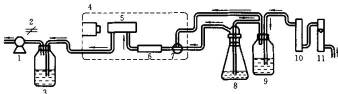
1—抽气泵;2—空气流量调节阀;3—含汞废气吸收器;4—测汞仪;5—光吸收池;6—干燥管; 7—三通阀;8—汞蒸气发生瓶;9—空气净化装置;10—活性炭吸收器;11—气体流量计
