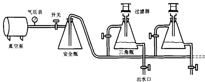
图 18 抽滤系统图
