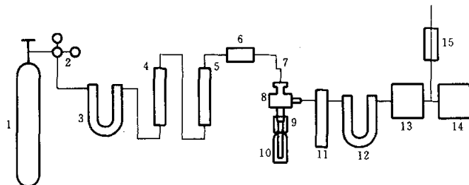
1—高纯氮气钢瓶;2—压力调节阀;3—活性碳 U 形管;4—5A 分子筛;5—碱石棉管;6—流量计; 7—不锈钢导管;8—聚四氟乙烯密封夹具;9—弹性胶管;10—安瓿瓶;11—盛盐酸羟胺溶液洗气瓶; 12—无水高氯酸镁;13—二氧化碳分析仪;14—记录仪;15—尾气流量计
