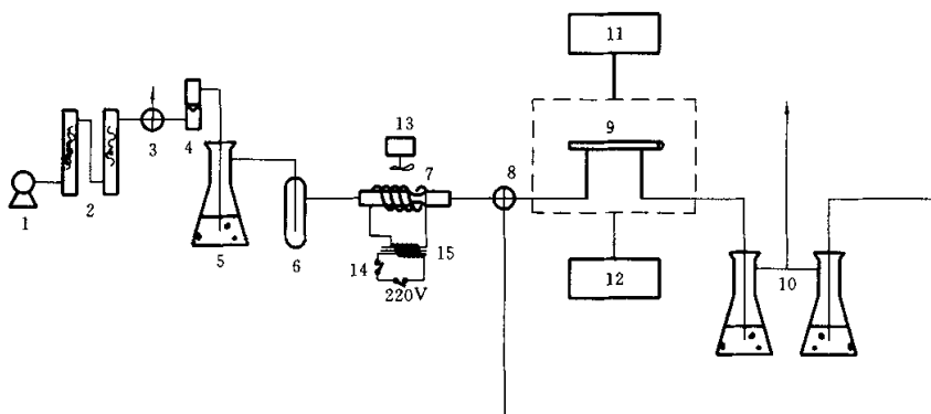
1—空气压缩机；2—气体净化装置；3—气体流量调节三通阀；4—转子流量计；5—反应瓶；6—缓冲瓶； 7—金捕集器；8—汞蒸气导入三通阀；9—测汞仪吸收池；10—尾气吸收瓶；11—记录仪；12—交流稳压器； 13—电吹风；14—金捕集器加热开关；15—调压变压器
