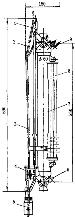
1—释放机构；2—活门；3—钢丝绳；4—夹紧装置；5—使锤； 6—气门；7—采水筒；8—温度表架；9—水咀
