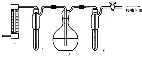
1—气体流量计；2—活芯气体采样管；3—汞蒸气发生瓶
