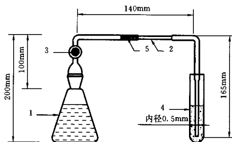
1—250 mL 锥瓶;2—乳胶管;3—乙酸铅棉花;4—吸收管;5—二甲基甲酰胺
