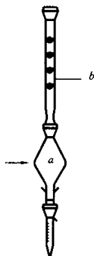
a—100 mL 锥形蒸馏瓶;b—内径 20×300 mm 分馏柱
